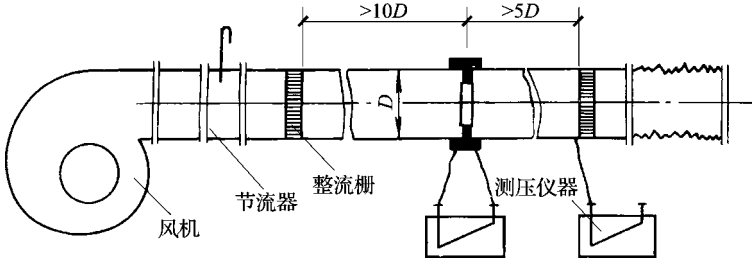
图 C.2.6-1 正压风管式漏风量测试装置
