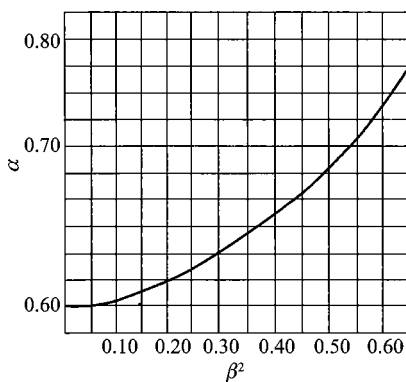
图 C. 2. 6-2 孔板流量系数图
