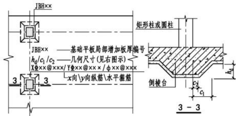
图7.2.4-1 倒棱台形增加板厚引注图示
