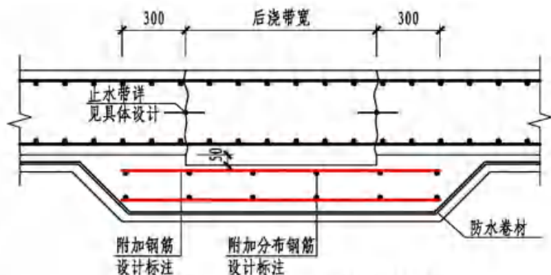
后浇带HJD下抗水压垫层构造
