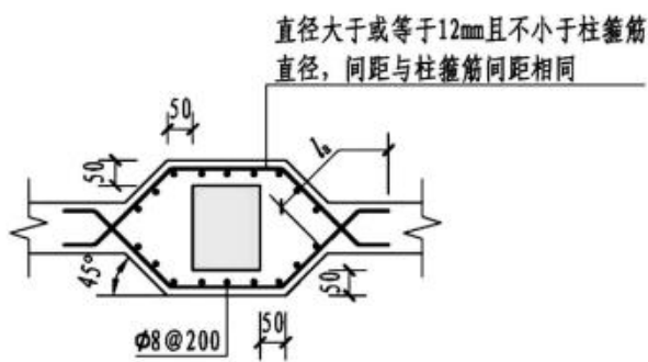
基础梁中心穿柱侧腋构造
