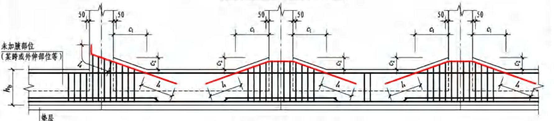
基础梁JL竖向加腋钢筋构造
