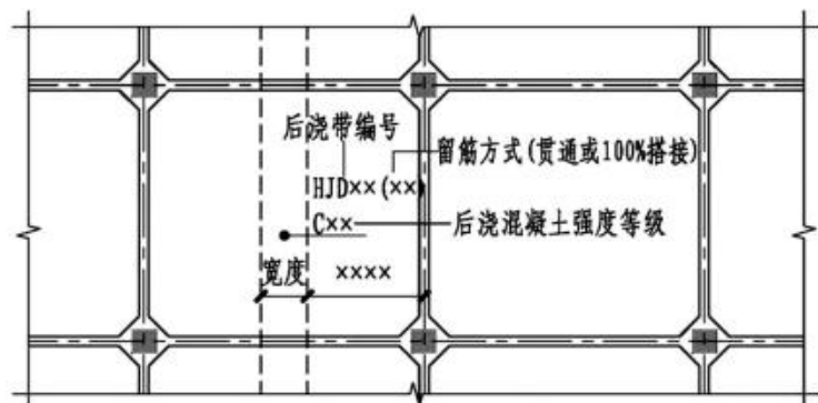
图7.2.2 后浇带HJD引注图示
