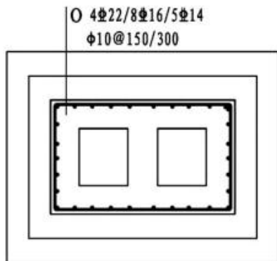
图2.3.2-14 双高杯口独立基础短柱配筋示意
