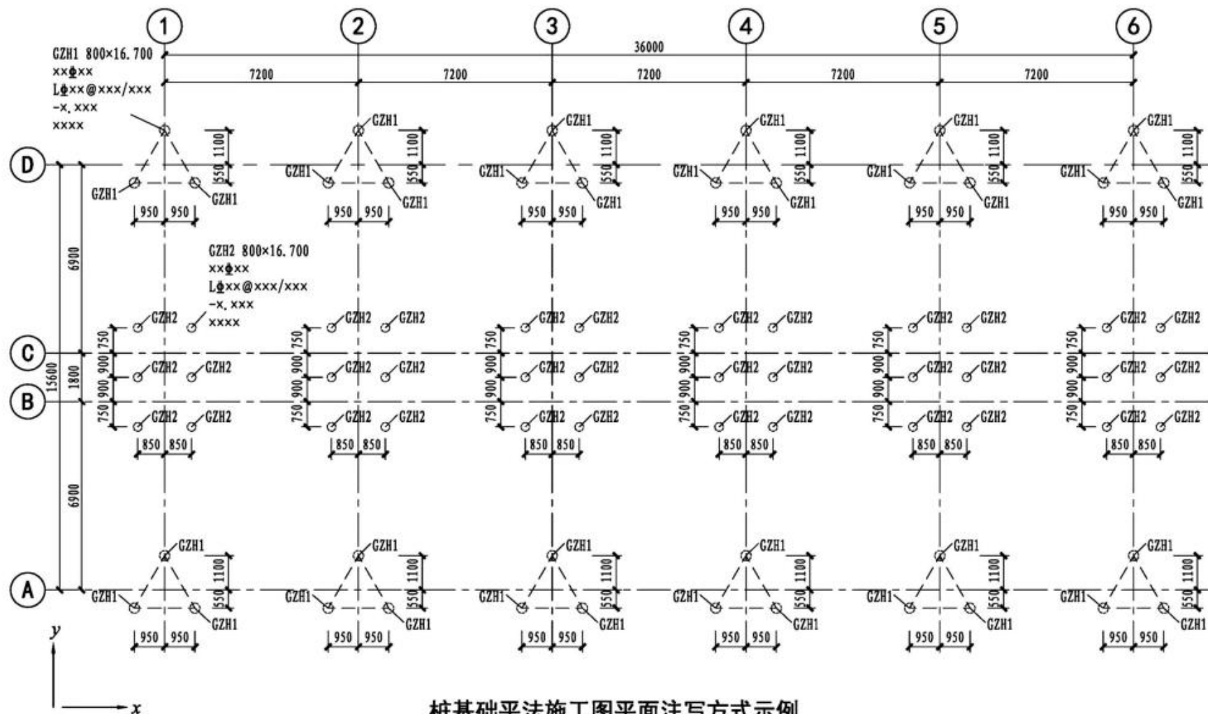
桩基础平法施工图平面注写方式示例
