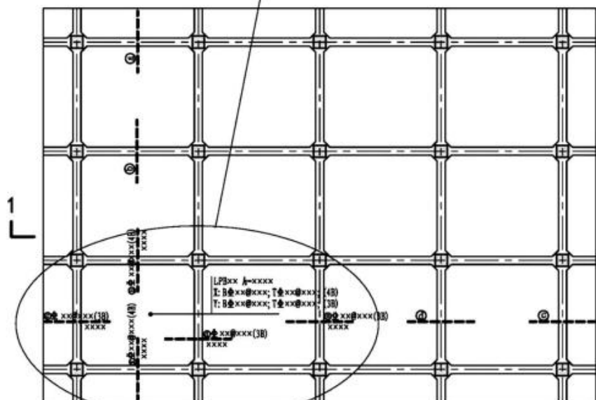
梁板式筏形基础平板LPB标注图示
