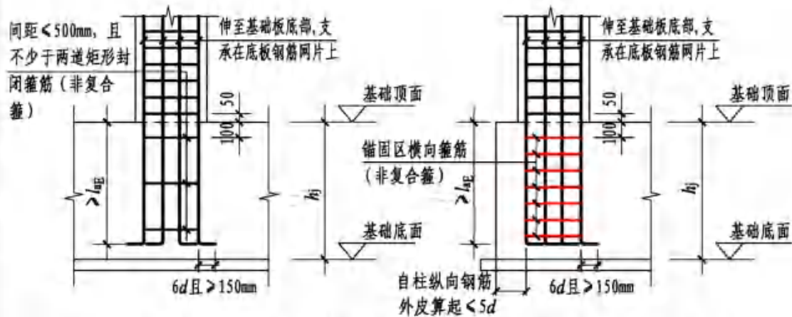
(a) 保护层厚度 > 5d ; 基础高度满足直锚 (b) 保护层厚度 < 5d ; 基础高度满足直锚
