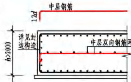
中层筋端头构造
