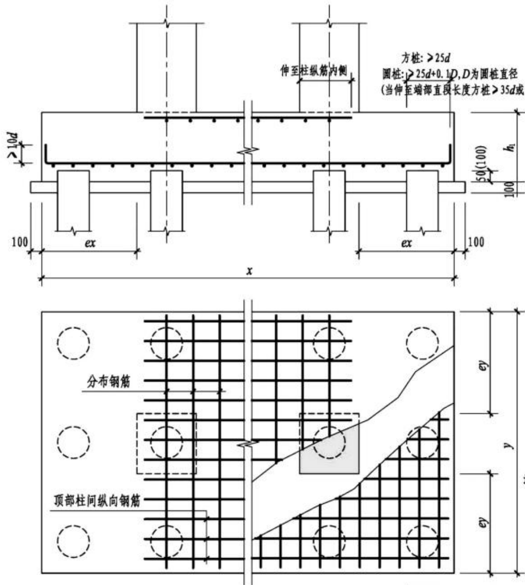
双柱联合承台底部与顶部配筋构造
