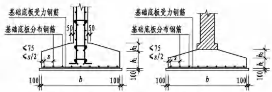
(剪力墙下条形基础截面)
