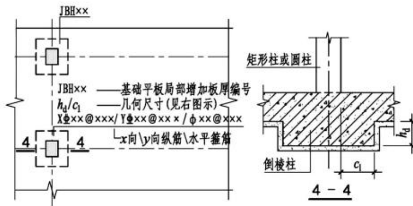
图7.2.4-2 倒棱柱形增加板厚引注图示
