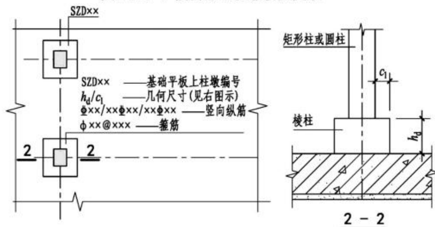
图7.2.3-2 棱柱形上柱墩引注图示
