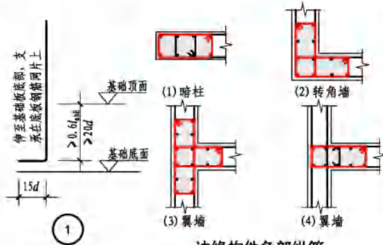
边缘构件角部纵筋
