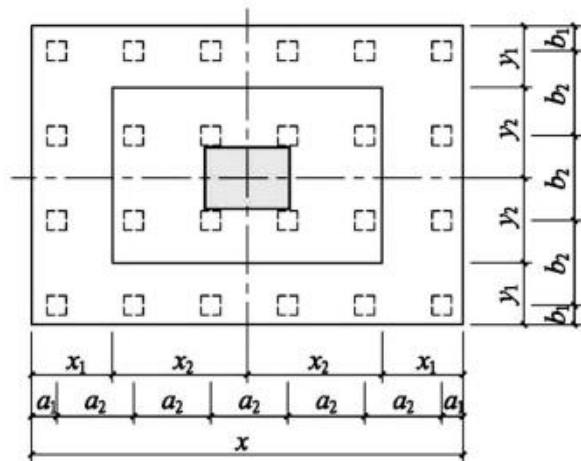
图6.6.3-1 矩形独立承台平面原位标注
