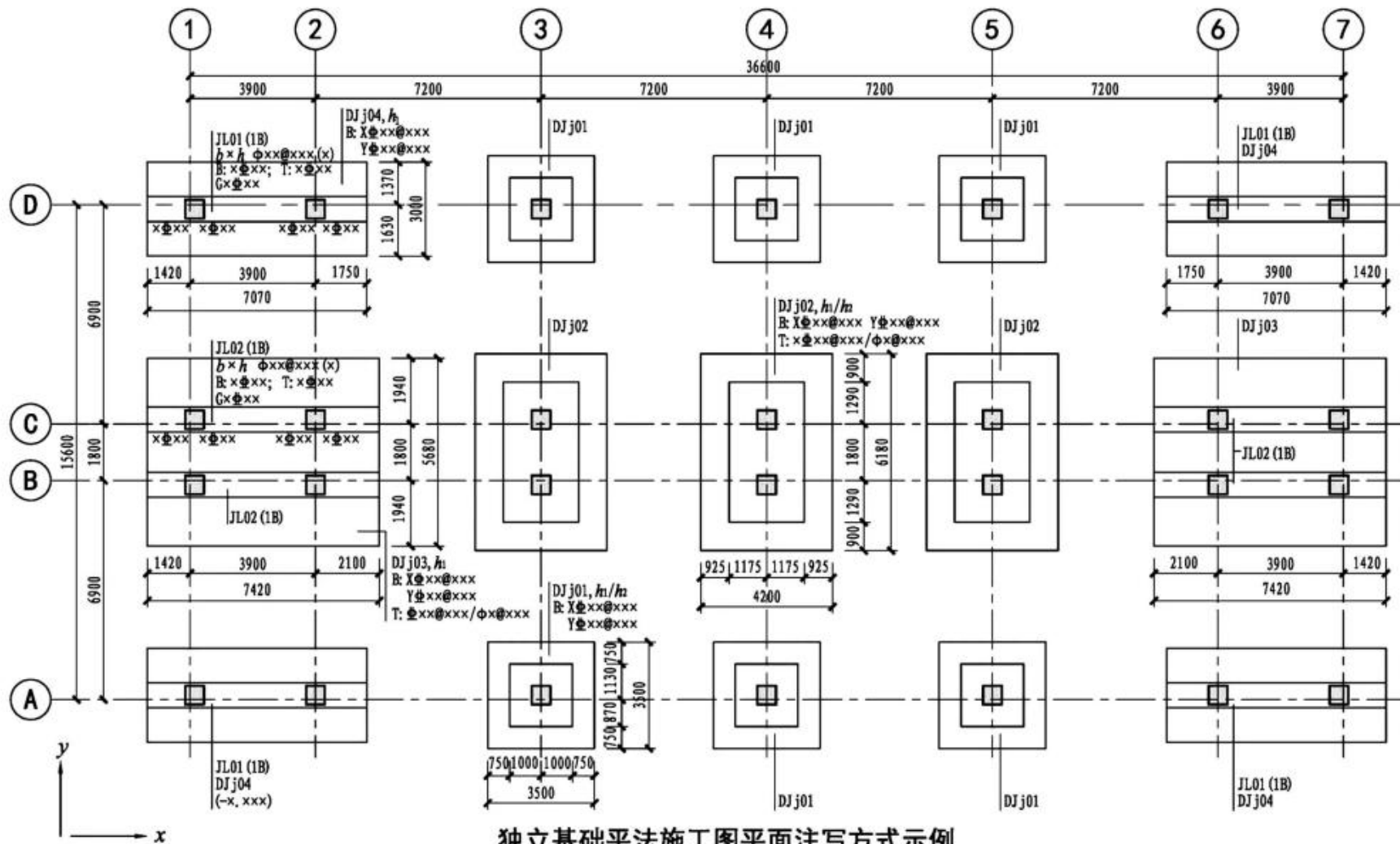
独立基础平法施工图平面注写方式示例
