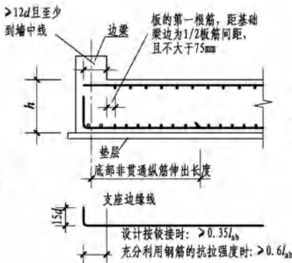
端部无外伸构造 (二)
