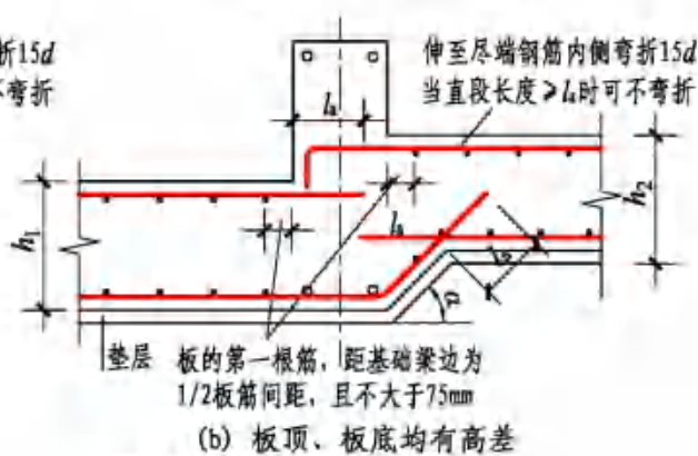
变截面部位钢筋构造
