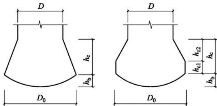
图6.2.2 扩底灌注桩扩底端示意
