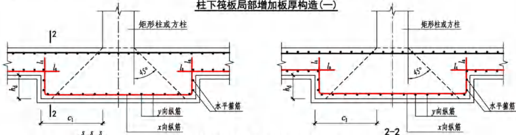
柱下筏板局部增加板厚构造(二)
