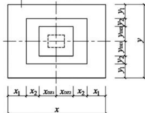
图2.3.4-2 带短柱独立基础平面注写方式设计表达示意
