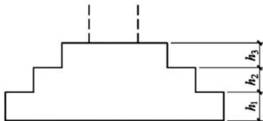
图2.3.2-1 阶形截面普通独立基础竖向尺寸
