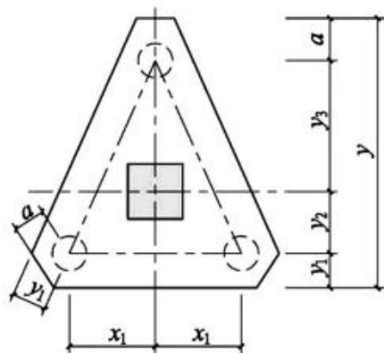
图6.6.3-3 等腰三桩独立承台平面原位标注
