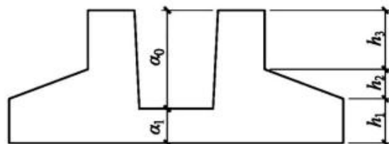
图2.3.2-8 锥形截面杯口独立基础竖向尺寸
