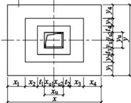
图2.3.5 杯口独立基础平面注写方式设计表达示意
