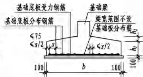
(坡形截面TJBp)
