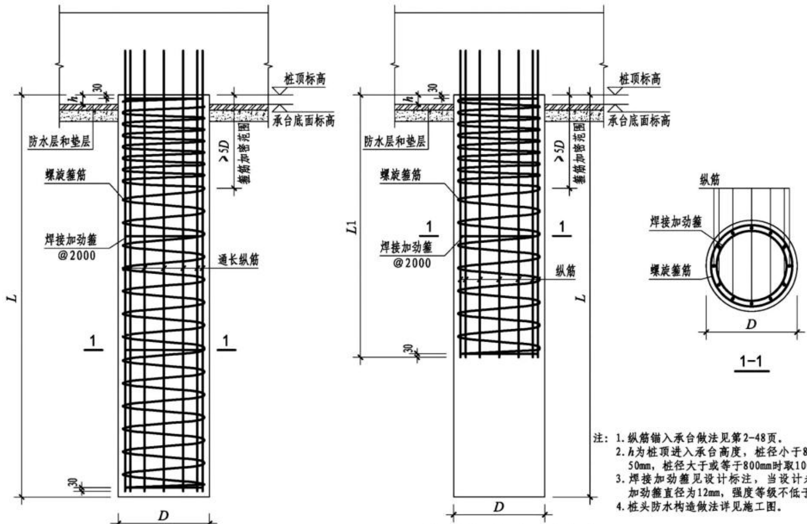
灌注桩部分长度配筋构造
