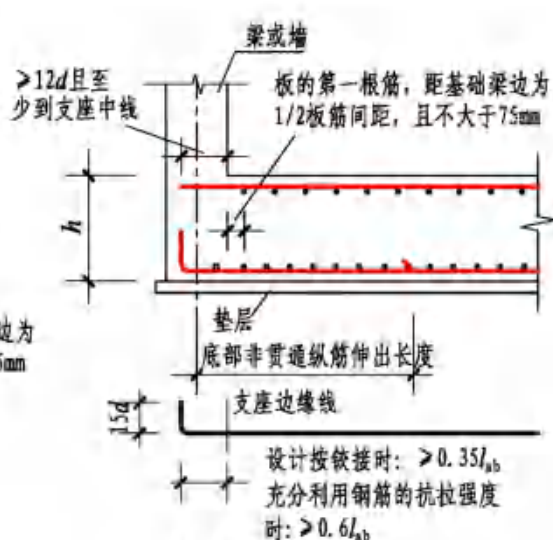
端部无外伸构造
