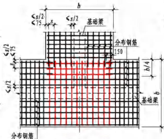
(b) 丁字交接基础底板
