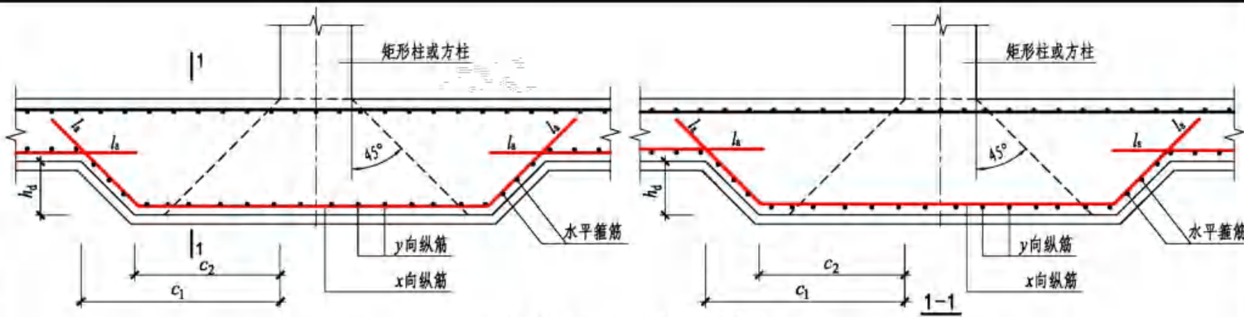
柱下筏板局部增加板厚构造(一)
