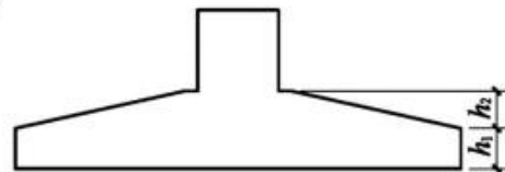
图3.5.2-1 条形基础底板坡形截面竖向尺寸
