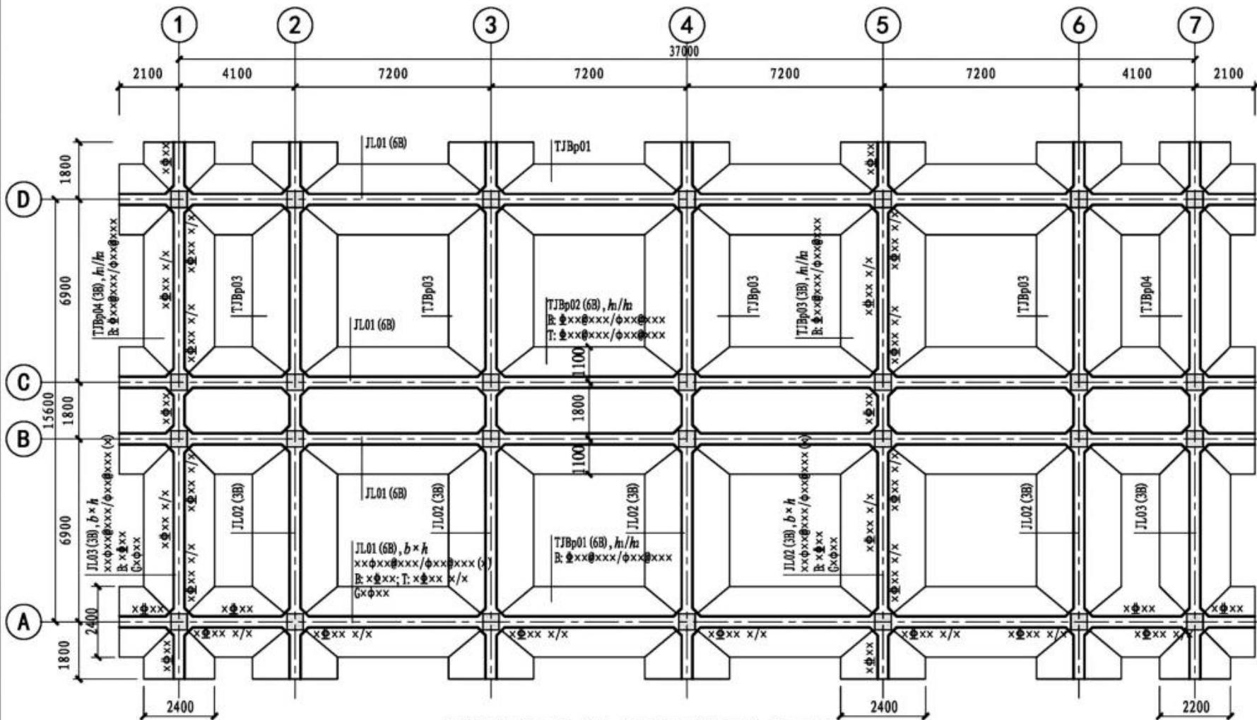
条形基础平法施工图平面注写方式示例
