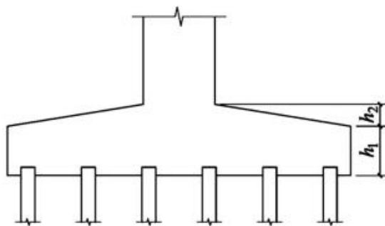
图6.6.2-3 锥形截面独立承台竖向尺寸
