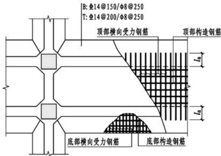
图3.5.2-4 双梁条形基础底板配筋示意
