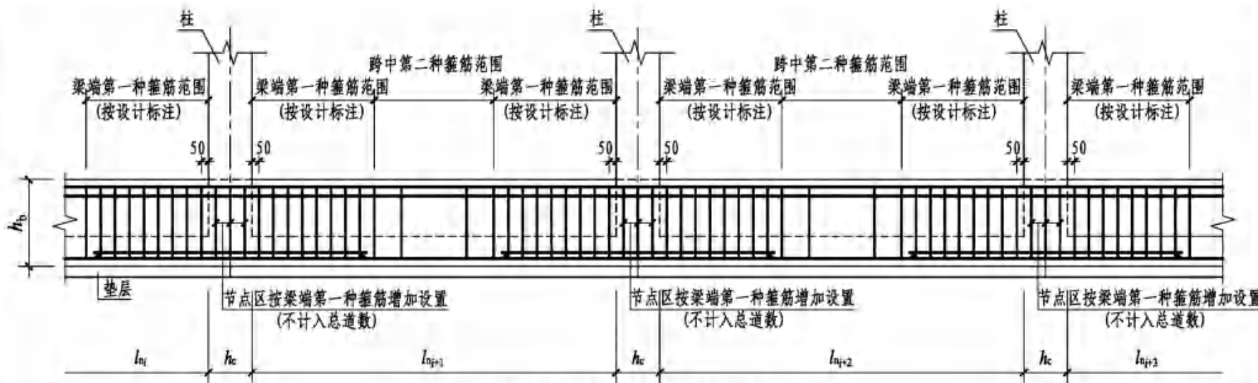
基础梁JL配置两种箍筋构造
