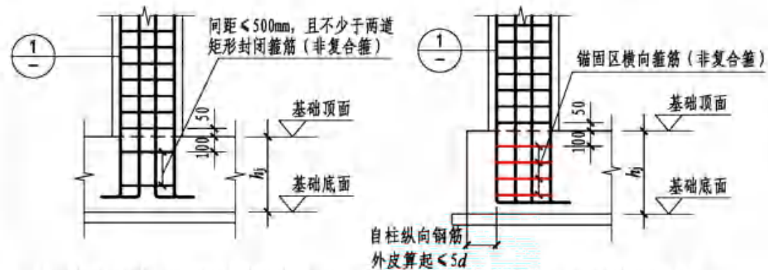
(c) 保护层厚度 > 5d ; 基础高度不满足直锚 (d) 保护层厚度 < 5d ; 基础高度不满足直锚
