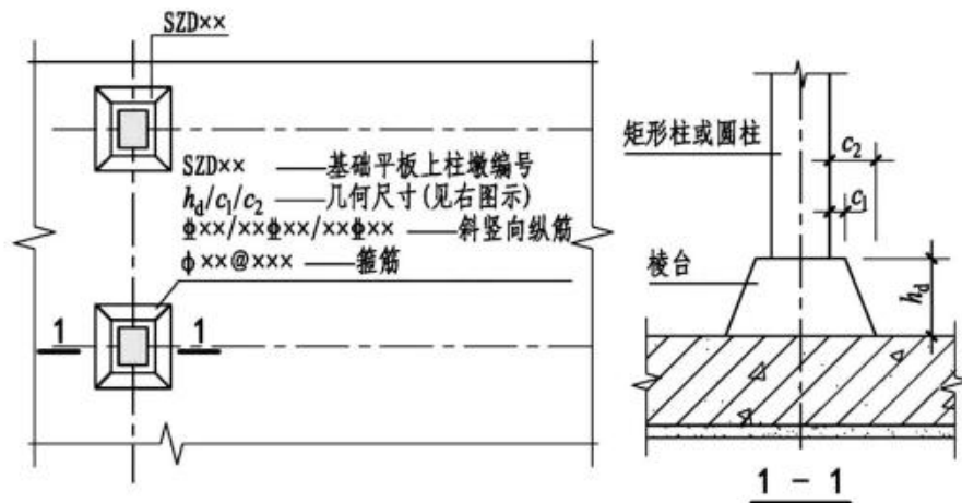
图7.2.3-1 棱台形上柱墩引注图示
