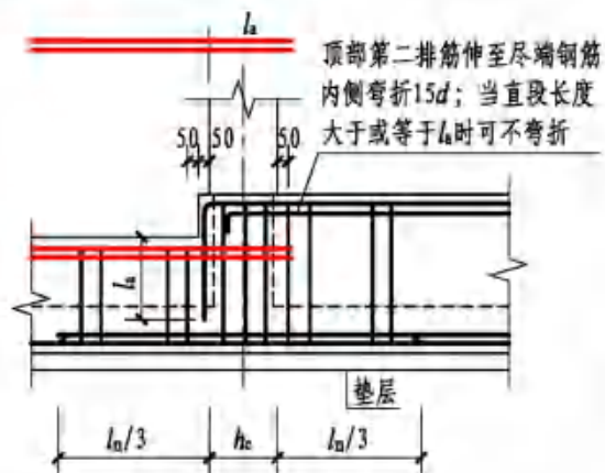
梁顶有高差钢筋构造
