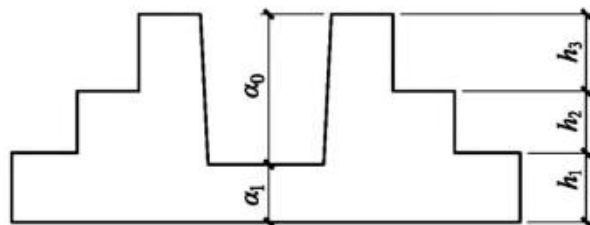
图2.3.2-4 阶形截面杯口独立基础竖向尺寸(一)
