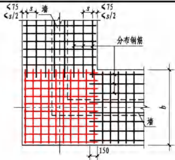
(a) 转角处墙基础底板
