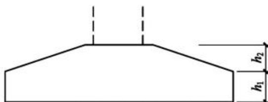
图2.3.2-3 锥形截面普通独立基础竖向尺寸
