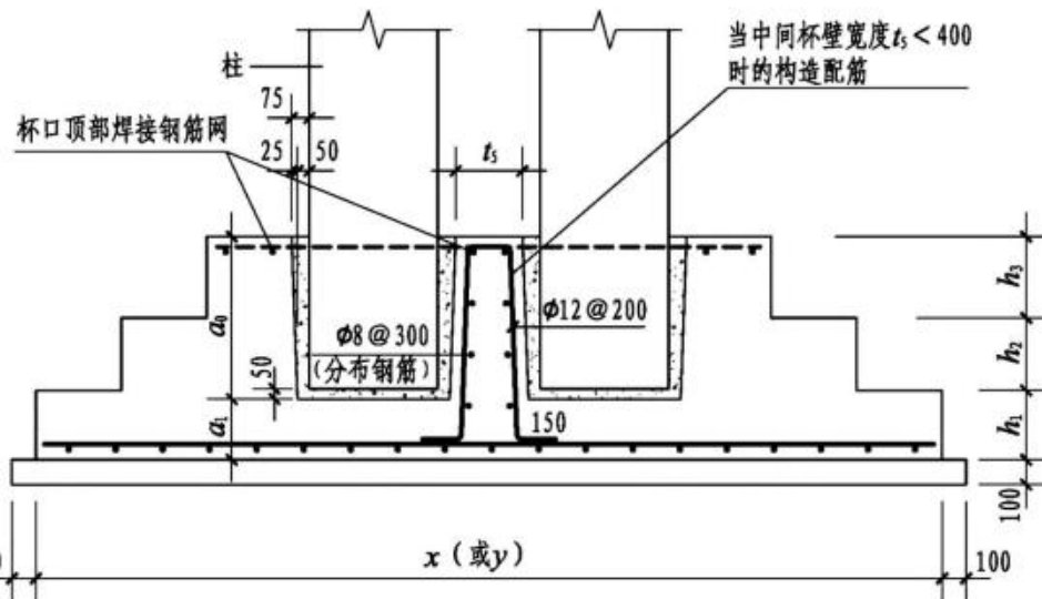
双杯口独立基础构造
