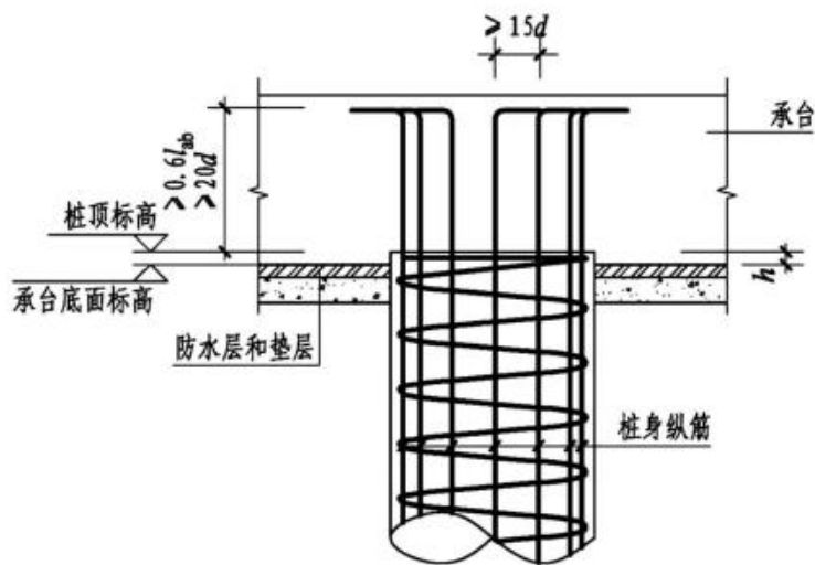
桩顶与承台连接构造 (二)
