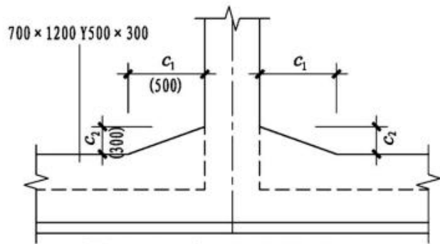
图3.2-1 竖向加腋截面注写示意
