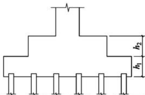
图6.6.2-1 阶形截面独立承台竖向尺寸
